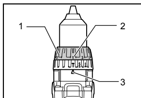
1. Bague de réglage 2. Graduation 3. Flèche
